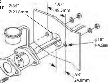
Figure 9 – Le support se monte de l'extérieur vers l'intérieur
